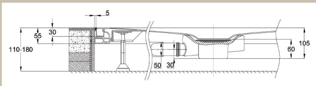
Wymiary montażowe z odpływem bocznym Montażni rozměry při bočním odtoku vody
