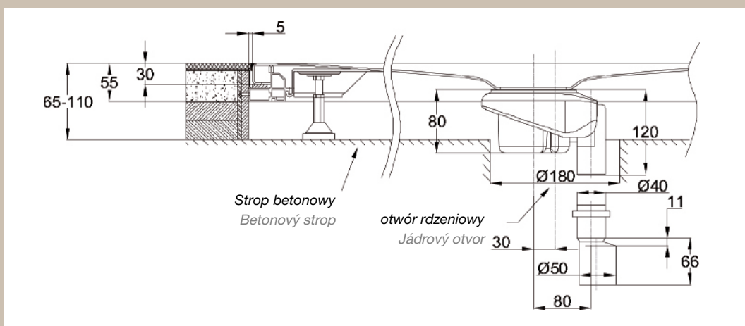
Wymiary montażowe z odpływem pionowym Montážni rozměry při svislém odtoku vody
